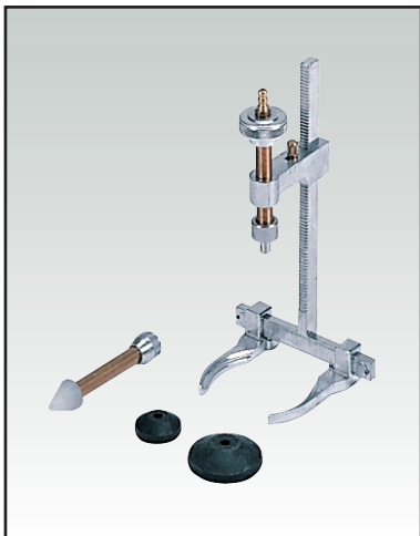
TAPPO UNIVERSALE W CON 3 TAMPONI CONICI UNIVERSAL PLUG W WITH 3 TAPERED PLUGS
